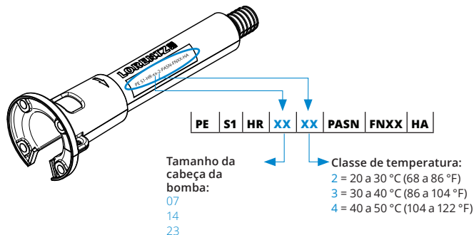
Figura 1: Nomenclatura da bomba
